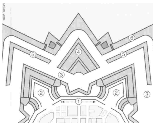
Fig. 4: Deel van een vestingsfront, aangelegd volgens het Nieuw-Nederlandse stelsel, eerste manier (NIMH): 1 courtine, 2 bastion, 3 gracht, 4 ravelijn, 5 covey-face, 6 enveloppe met wapenplaatsen
